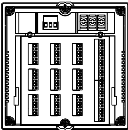
压紧接线端子后的仪表后视图
