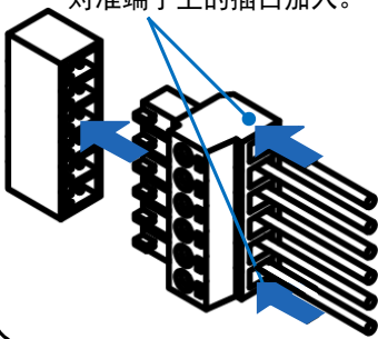
压紧接线端子后的仪表后视图
